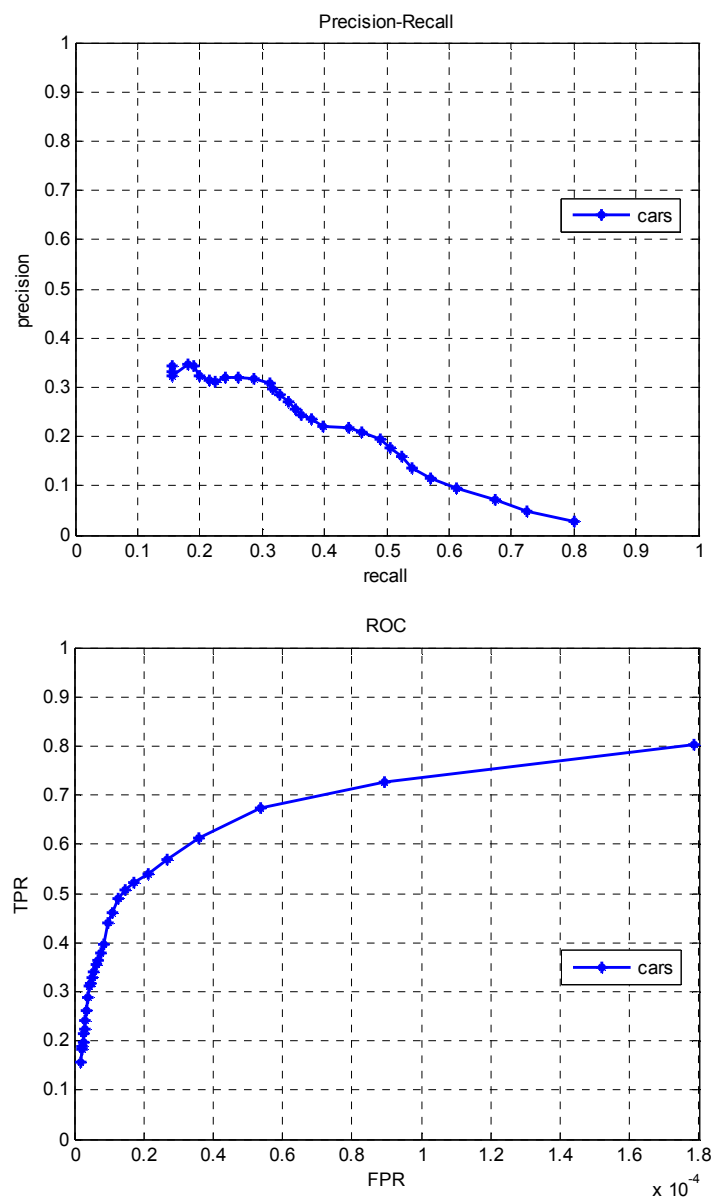
Σχήμα 4.19 - Καμπύλες ακρίβειας–επανάληψης και ROC του συνδυασμού των ανιχνευτών για αυτοκίνητα
