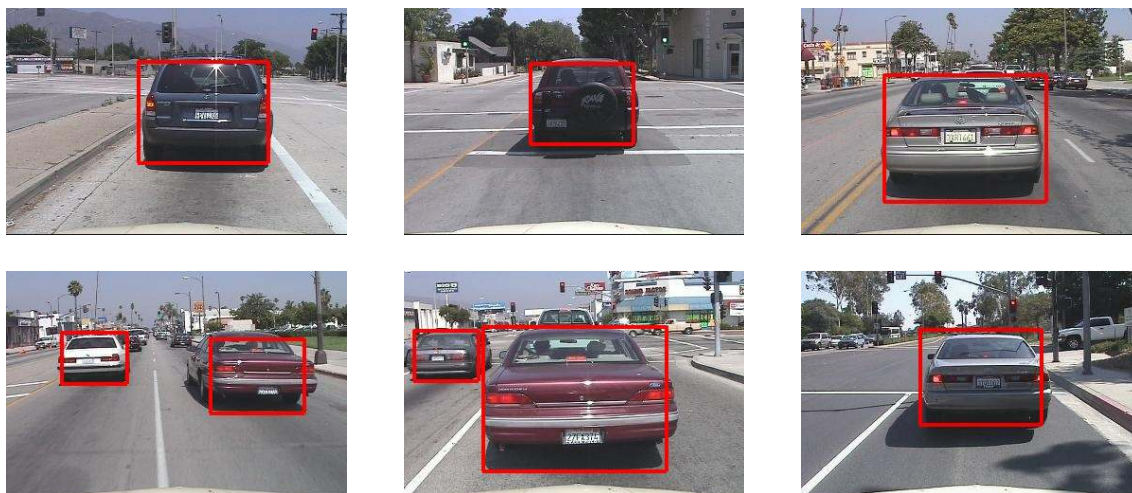
Σχήμα 4.16 - Αποτελέσματα της ανίχνευσης για την εμπρός και πίσω όψη αυτοκινήτων στο δεύτερο σύνολο εικόνων δοκιμής.
