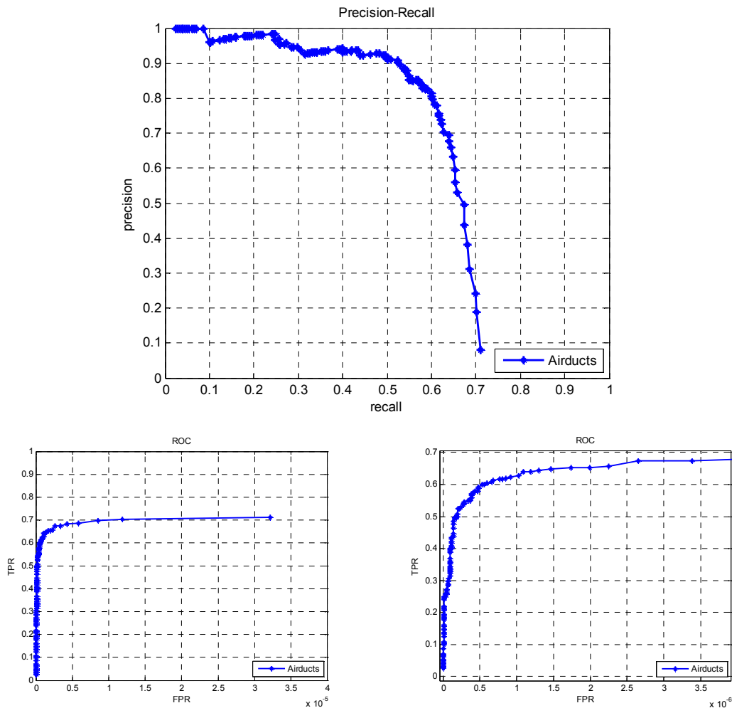
Σχήμα 4.5 - Καμπύλη ακριβείας-επανάληψης και ROC του ανιχνευτή για τους αεραγωγούς αυτοκινητών
