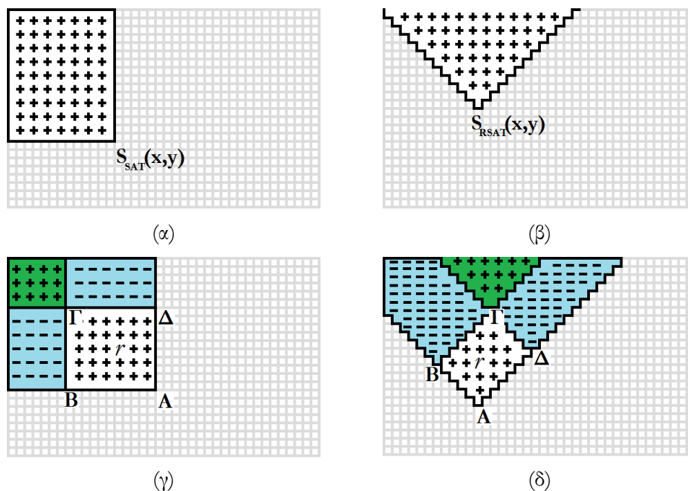
Σχήμα 2.2 - Οι πίνακες που βοηθούν στο γρήγορο υπολογισμό των χαρακτηριστικών. α) Πίνακας Προστιθέμενου Εμβαδού S_{SAT} , β) Περιστραμμένος Πίνακας Προστιθέμενου Εμβαδού S_{RSAT} , γ) Υπολογισμός κατακόρυφου ορθογωνίου, δ) Υπολογισμός περιστραμμένου ορθογωνίου
