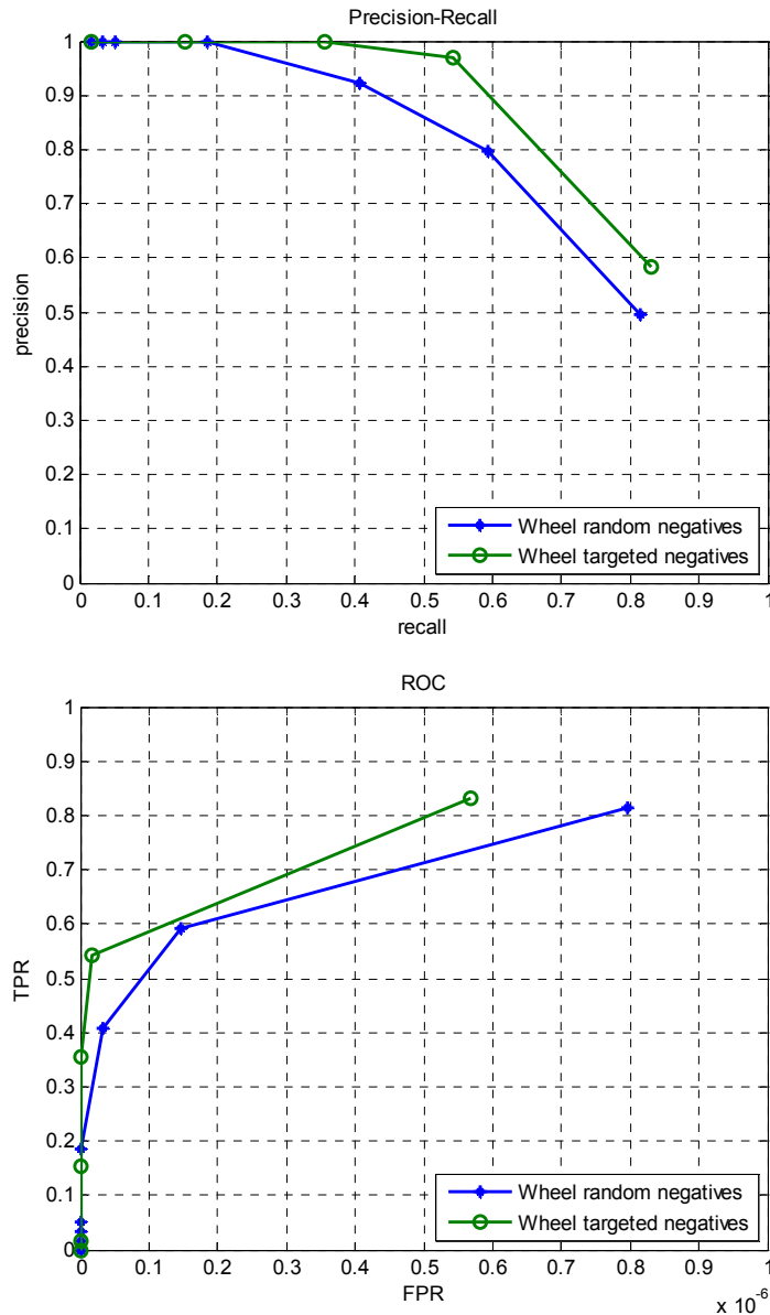
Σχήμα 4.2 - Καμπύλες ακρίβειας-επανάλληξης και ROC των ανιχνευτών για τα τιμόνια αυτοκινήτων
