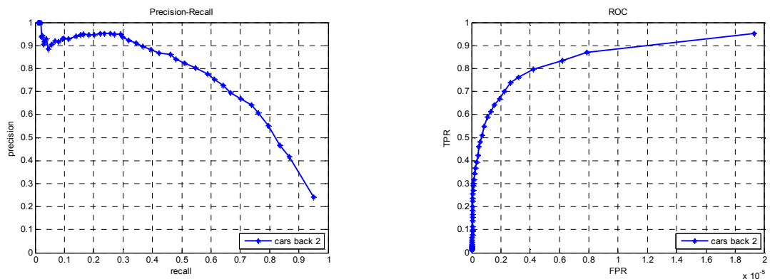
Σχήμα 4.14 - Καμπύλες ακριβείας–επανάκλησης και ROC του ανιχνευτή εμπρός και πίσω όψης αυτοκινήτων. α) Αποτελέσματα από την πρώτη ομάδα εικόνων, β) αποτελέσματα από τη δεύτερη ομάδα εικόνων
