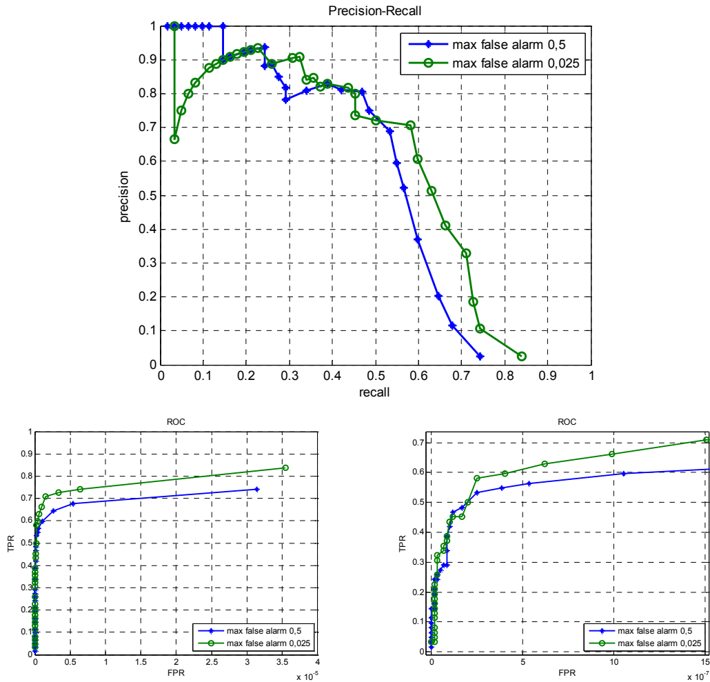
Σχήμα 4.8 - Καμπύλες ακρίβειας–επανάληψης και ROC των ανιχνευτών για τους μοχλούς ταχυτήτων
